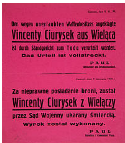
Fragment ekspozycji
